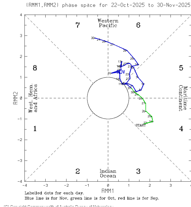
Gambar 7. Fase MJO Bulan November 2025
