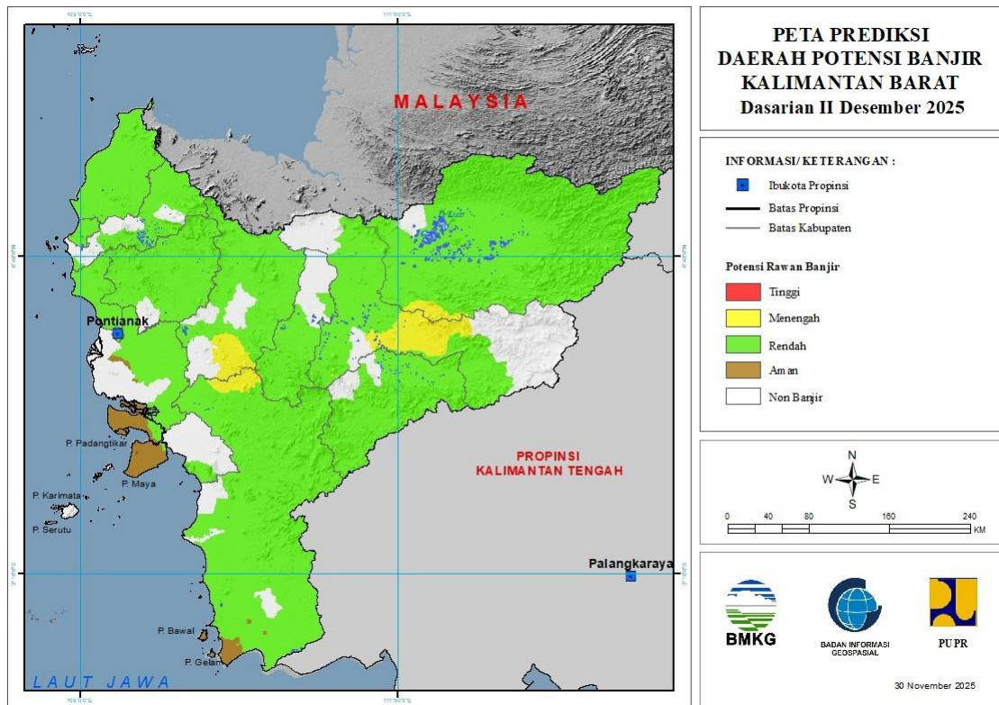
Gambar 16. Peta Prediksi Daerah Banjir Wilayah Kalimantan Barat Desember Dasarian 2
