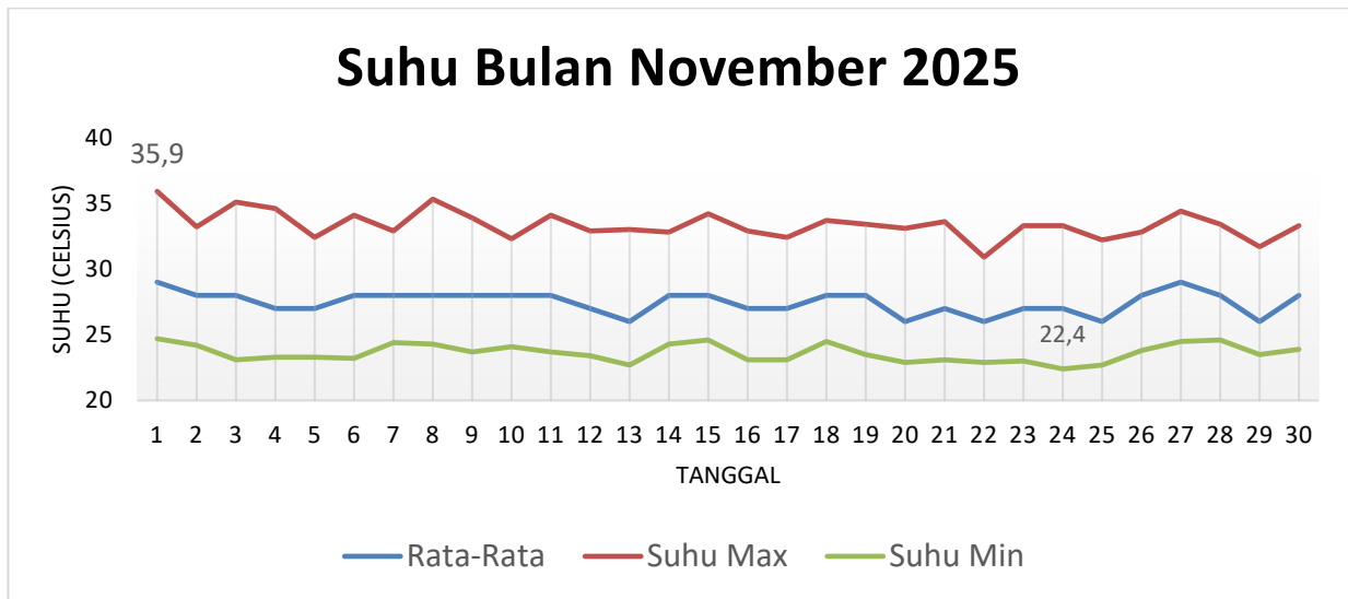
Gambar 12. Grafik Suhu Udara Bulan November 2025
