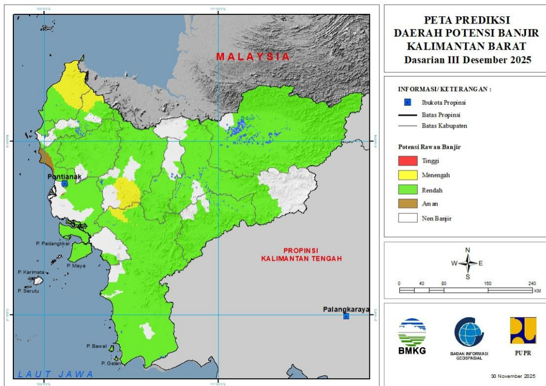
Gambar 17. Peta Prediksi Daerah Banjir Wilayah Kalimantan Barat Desember Dasarian 3
