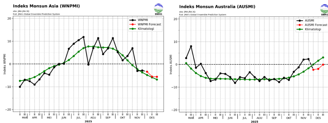
Gambar 9. Grafik Pergerakan Index Monsoon
