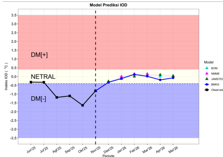
Gambar 4. Prediksi IOD Oleh Institusi Internasional dan BMKG
