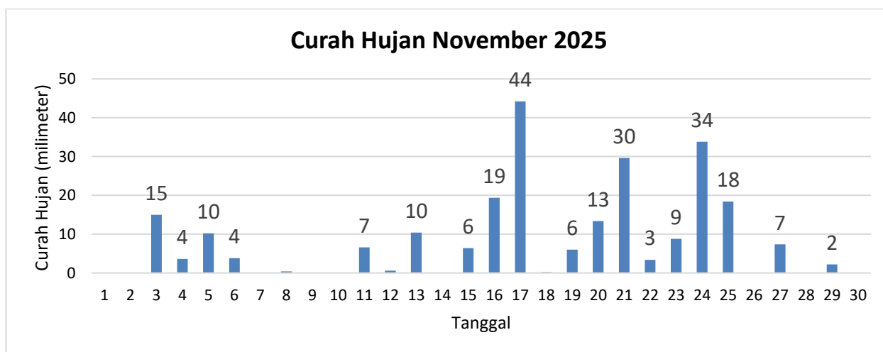
Gambar 10. Grafik Curah Hujan Bulan November 2025
