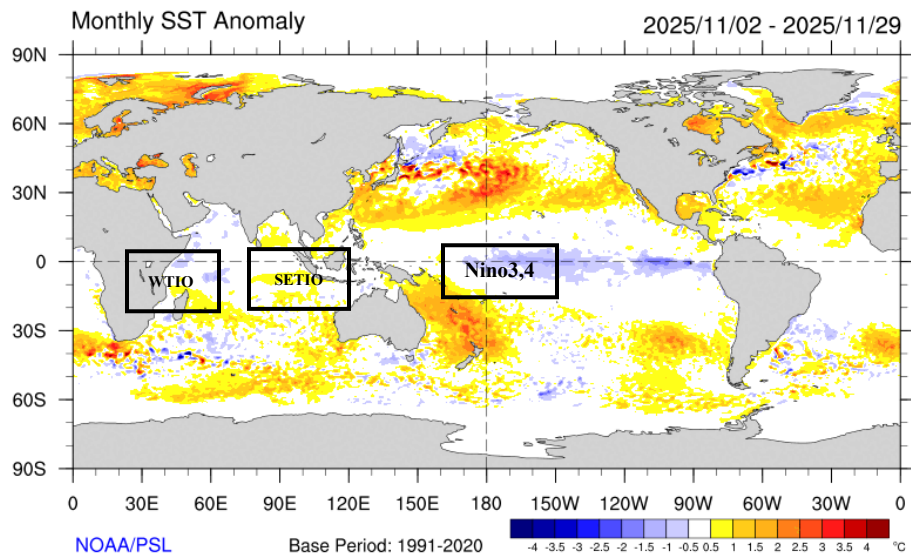
Gambar 2. Anomali Suhu Muka Laut Bulan November 2025
