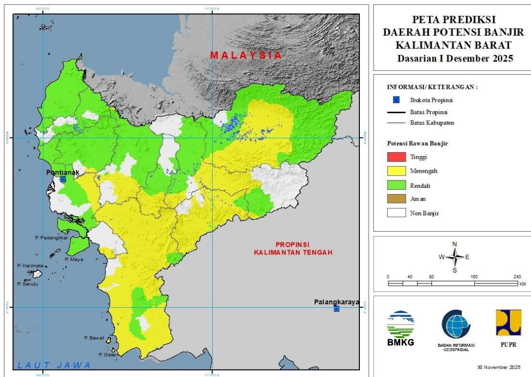
Gambar 15 Peta Prediksi Daerah Banjir Wilayah Kalimantan Barat Desember Dasarian 1
