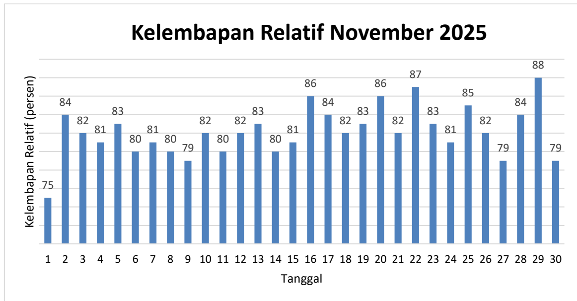
Gambar 13. Grafik kelembapan udara relatif bulan November 2025
