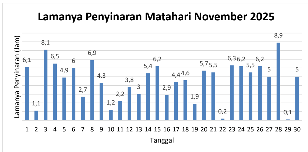
Gambar 14. Grafik Lama Penyinaran Matahari Bulan November 2025
